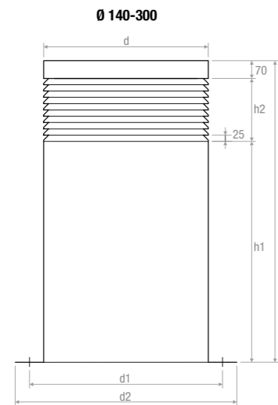
Versione con silenziatore Version with sound attenuator
