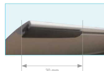
Battute di serie come da foto Series swabs as picture
