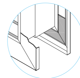
PARTICOLARE INSERIMENTO CONTROCORNICE PARTICULAR INSERTION COUNTERFRAME
