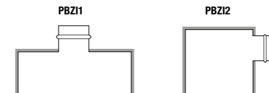
Plenum isolato esternamente spessore 6 mm Plenum externally insulated thickness 6 mm
