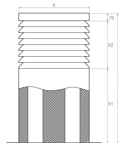
Versione con silenziatore Version with sound attenuator
